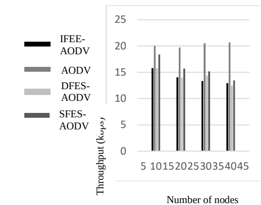
(شکل-۱۲): مقایسهٔ بازده IFEE-AODV با DFES-AODV ، AODV و SFES-AODV
