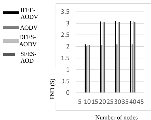
(شکل-۱۴): مقایسهٔ معیار FND پروتکل IFEE-AODV با DFES-AODV ، AODV و SFES-AODV
