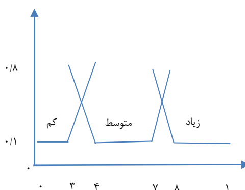
(شکل-۶): تابع عدم عضویت انرژی باقیمانده (Figure-6): Non-membership function of remaining energy
