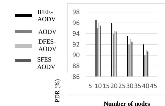
(شکل-۱۰): مقایسهٔ نرخ تحویل بسته IFEE-AODV با DFES-AODV ، AODV و SFES-AODV
