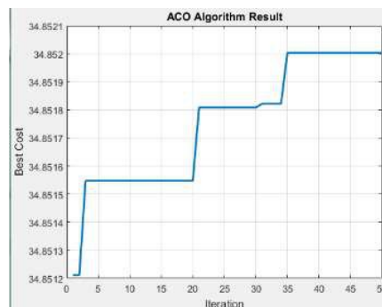
(شکل-۵): نمودار افزایش PSNR در تکرارهای مختلف اجرای الگوریتم ACO در تصویر لنا
