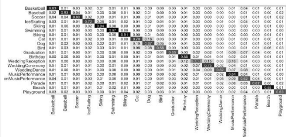
(شکل-۳): ماتریس ابهام طبقه‌بندی روش پیشنهادی بر روی مجموعه داده CCV.
