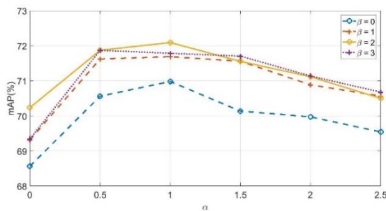
(شکل-۲): دقت تشخیص وقایع نسبت به پارامترهای تنظیم برای توصیف‌گرهای هزار بُعدي و هشت خوشه روی مجموعه داده CCV.
