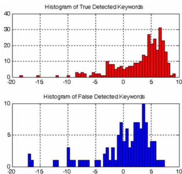
(شکل ۸): هیستوگرام امتیاز اطمینان نرمالیزه شده کلیدواژه‌های درست (شکل بالا) یا غلط (شکل پایین)
