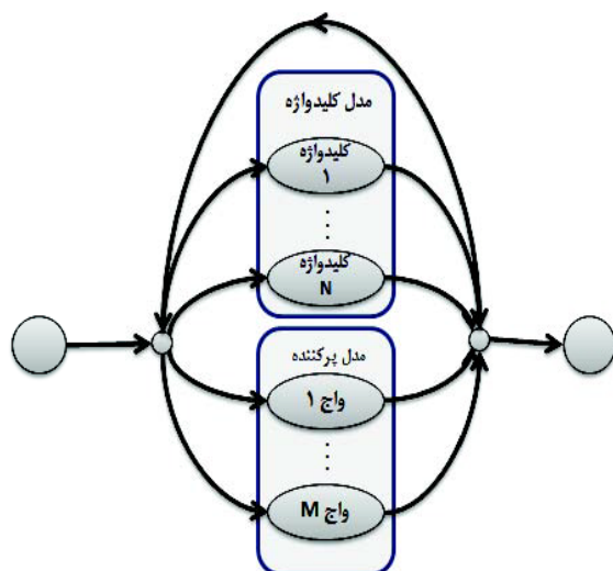
(شکل ۲): مدل شبکه کلمات (Net1) متشکل از N مدل کلیدواژه و M مدل پرکننده برای تولید رشته خروجی متناظر با سیگنال گفتار ورودی شامل کلیدواژه‌ها و مدل‌های پرکننده
