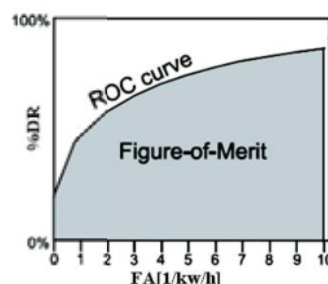
شکل ۴- نمایش منحنی ROC (Szoke et al., 2010).
