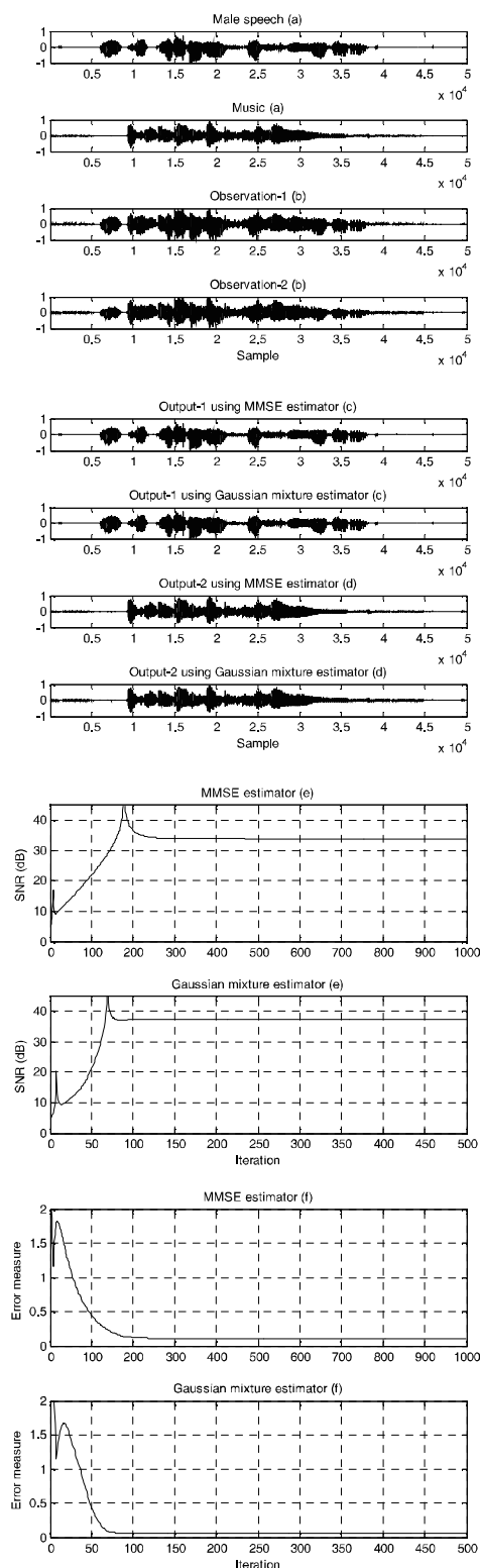
(شکل ۷: (a) منابع اولیه موسیقی و گوینده مرد، (b) مشاهدات، (c و d) مقایسه سیگنال‌های خروجی الگوریتم با دو تخمین زن، (e و f) مقایسه مقدار SNR و معیار خطای خروجی‌های الگوریتم با دو تخمین زن)
