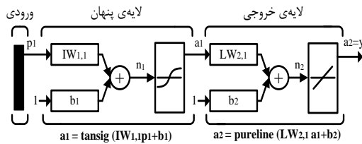
(شکل-۶): ساختار شبکه عصبی NN_P. (Figure-6): The Structure of Neural Network NN_P.
