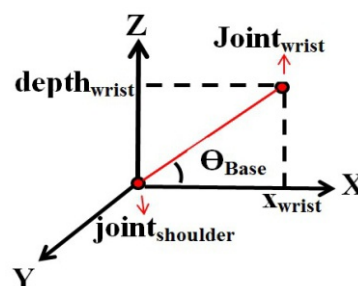
(شکل-۱۷): به‌دست‌آوردن \theta_{\text{Base}} در محور مختصات X-Z
