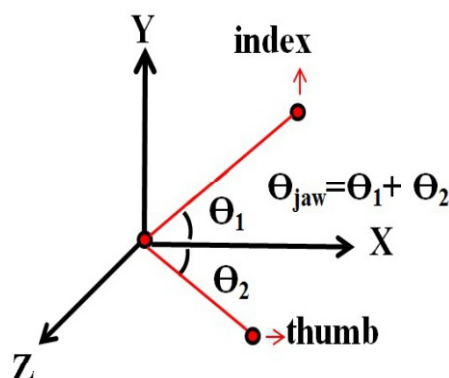
(شکل-۸): محاسبه مقدار باز شدن انگشتان از هم
