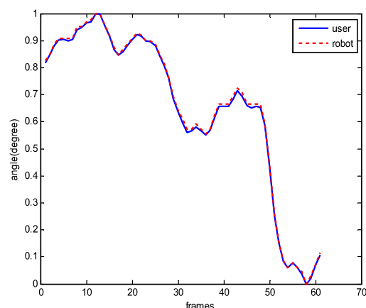
(شکل-۲۵): مقایسه تغییرات زاویه مجری نهایی برای کاربر و ربات
