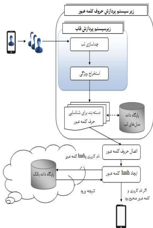
(شکل-۵): معماری سامانه پیشنهادی (Figure-5): The proposed system architecture
