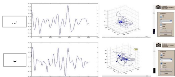
(شکل-۸): نمودار سیگنال‌های ABR و فضای فاز نمونه‌های ۲
