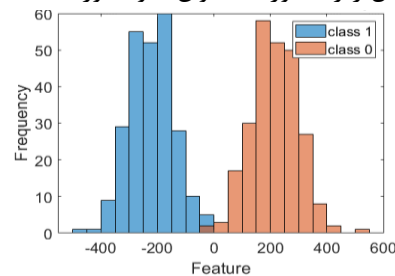
(شکل-۱۳): هیستوگرام ضرایب صفر و یک با L=6, M=1 ,
