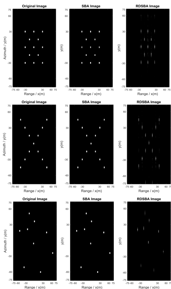
(شکل-۱۳): مقایسه تصاویر بازسازی‌شده مختلف توسط دو روش SBA و RDSBA.
