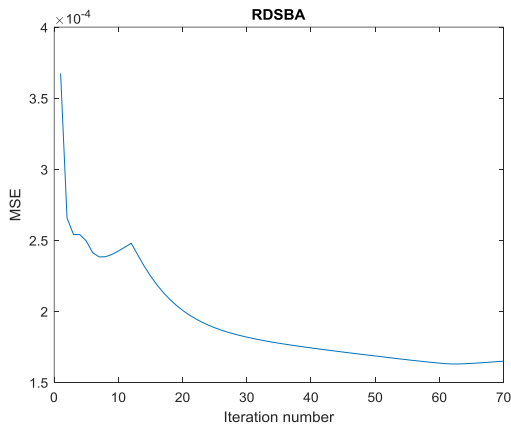
(شکل-۸): MSE حاصل در هر تکرار برای روش RDSBA با 63% داده، SNR=15dB و حضور خطای فاز.
