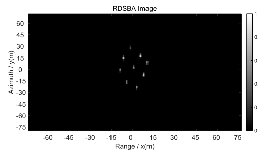
(شکل-۶): تصویر حاصل از روش پیشنهادی RDSBA با 63% داده، SNR=15dB و حضور خطای فاز.
