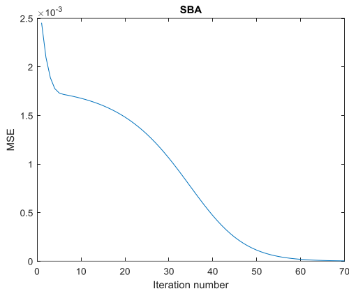
(شکل-۵): MSE حاصل از روش پیشنهادی RDSBA با 63% داده، SNR=15dB و حضور خطای فاز.
