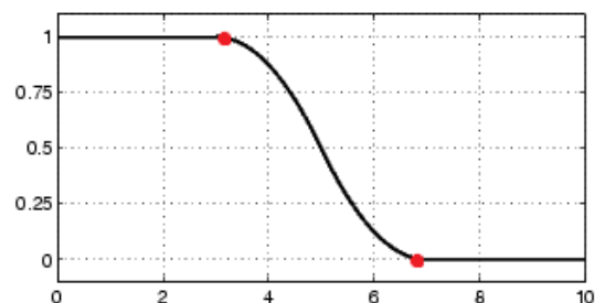
(شکل-۴): تابع عضویت zmf برای متغیر زبانی low (Figure-4): Zmf membership function for low linguistic variable
