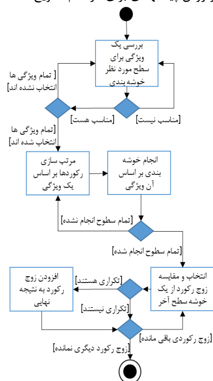
(شکل ۱-۱): نمودار فعالیت فرآیند تشخیص تکراری (Figure-1): Activity diagram of duplicate detection process
