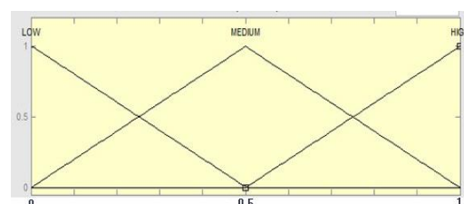
(شکل ۳): تابع عضویت متغیرهای سامانه فازی پیشنهادی (Figure-3): The Variables' membership function of the proposed fuzzy system
