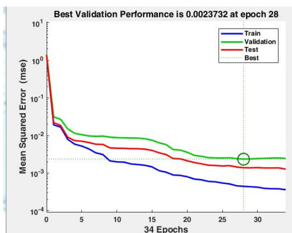
(شکل - ۲۳): نمودار همگرایی شبکه عصبی برای شرکت
