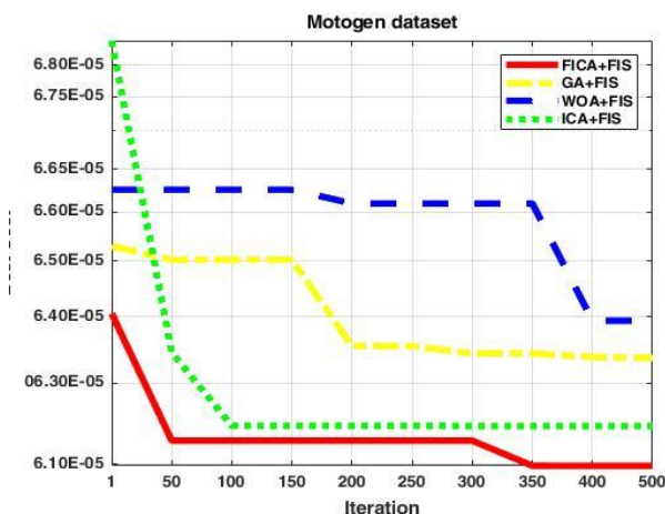
(شکل - ۱۸): نمودار همگرایی الگوریتم های گروه اول
