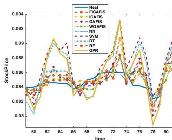
(شکل ۱۰-): نمودار مقایسه قیمت واقعی و پیش‌بینی‌شده
