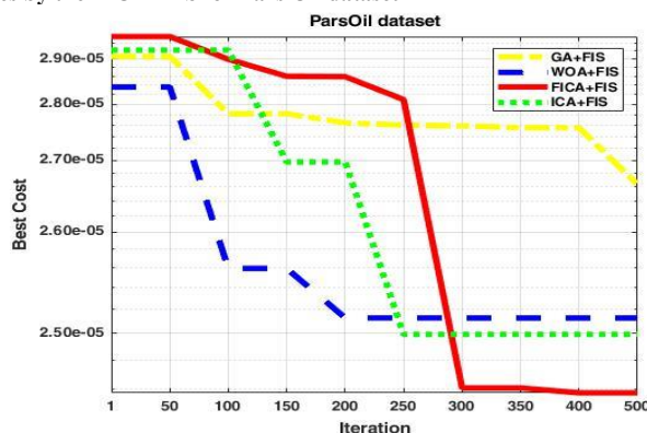
(شکل ۸): نمودار هم گرایی الگوریتم های گروه اول
