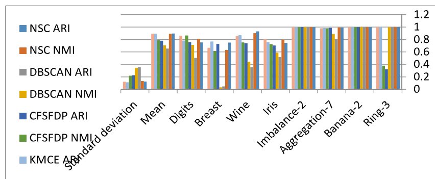
(شکل-۱۲): مقایسه با الگوریتم‌های خوشه‌بندی "قوی"
