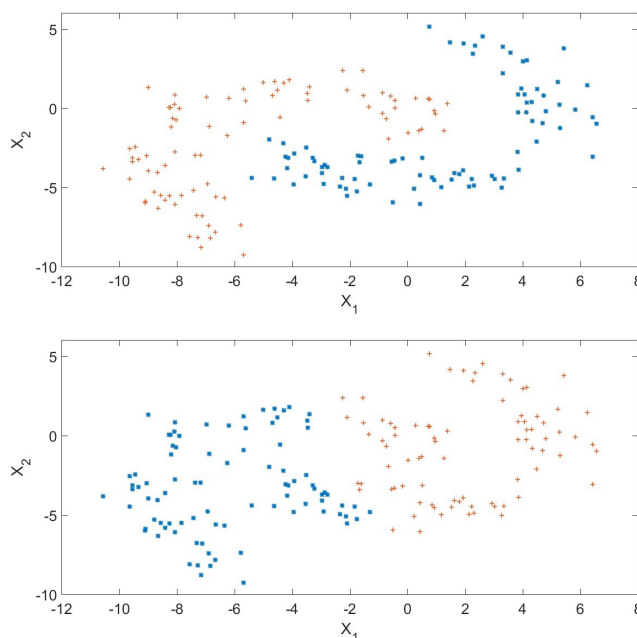
(شکل-۴): (الف) یک مجموعه داده و برچسب‌های خوشه واقعی (بالا). (ب) نتیجه اعمال الگوریتم خوشه‌بندی cmeans فازی (پایین). (Figure-4): (a) A dataset and true cluster labels (high). (B) The result of the fuzzy cmeans clustering algorithm (bottom).
