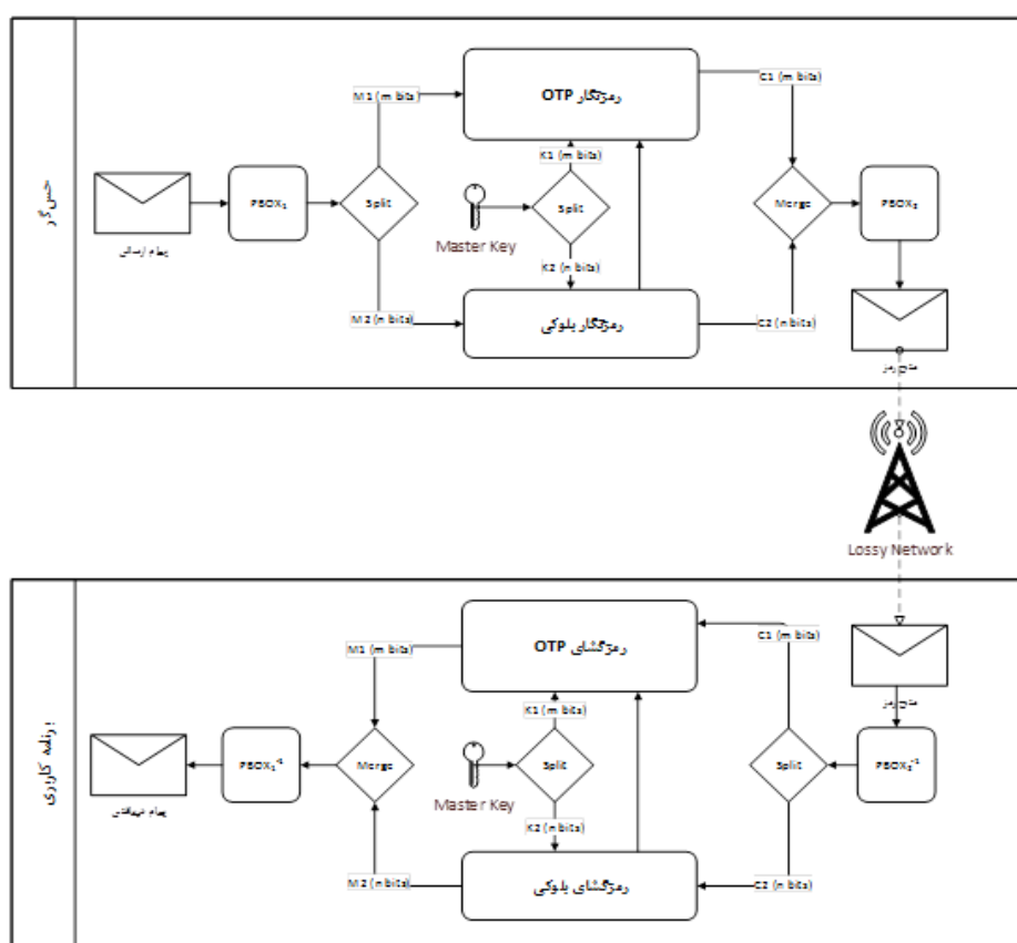
(شکل-۷): معماری کلی رمزنگار در حالت کاری صفر (Figure-7): General cryptographic architecture in zero working mode
