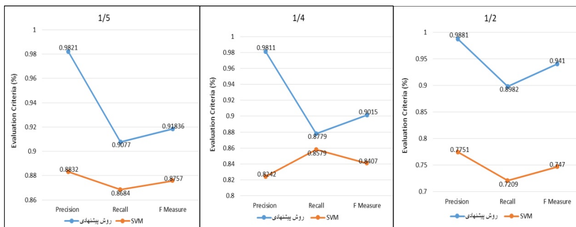
(شکل-۲): ارزيايى روش ها بر روى مجموعه داده Reuters 21578 با ۱/۵، ۱/۴ و ۱/۲ ويژگيهاى انتخابى از كل ويژگيها (Figure-2): Evaluation of Methods on the Reuters 21578 dataset with 1.2, 1.4 and 1.5 Features Selected from all Features
