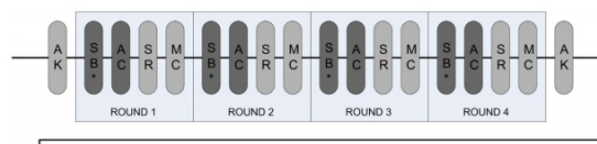
(شکل-۲): الگوریتم رمزنگاری Zorro (Figure-2): Zorro cipher algorithm
