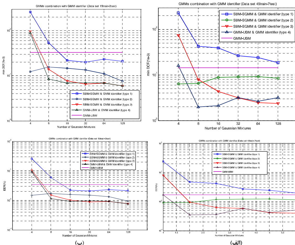
شکل (۷): عملکرد شناسایی کننده GMM به عنوان پردازشگر پسین در حوزه‌ی امتیازها (الف) ۴۵ ثانیه آموزش، ۷ ثانیه آزمون (ب) ۱۵ ثانیه آموزش، ۳ ثانیه آزمون (بالا نمودار min. DCF و پایین نمودار EER)
