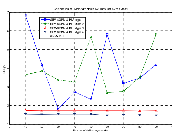
شکل (۶): عملکرد شبکه‌ی عصبی به عنوان پردازشگر پسین در حوزه‌ی امتیازها (الف) ۴۵ ثانیه آموزش، ۷ ثانیه آزمون (ب) ۱۵ ثانیه آموزش، ۳ ثانیه آزمون (بالا نمودار min. DCF و پایین نمودار EER)
