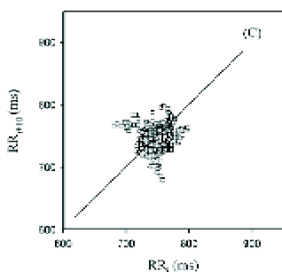
شکل (۴): نمودار پوآنکاره سیگنال RRI مربوط به سطح استرس (A) کم، (B) متوسط، (C) زیاد
