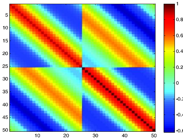
(شکل ۳) نمایش ماتریس همبستگی یک مخلوط ساده. خطوط اریب متناظر با همبستگی‌های فضایی در بلوک‌های غیرقطری قابل مشاهده، اما غیرمتمم‌گرا.
