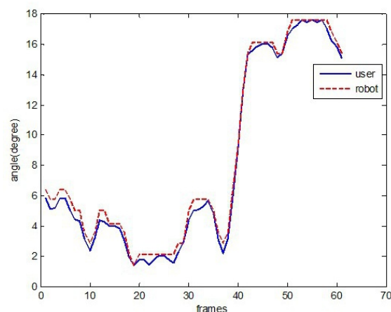
(شکل-۲۴): مقایسه تغییرات زاویه آرنج برای کاربر و ربات (Figure-24): changes of elbow angle for user and robot
