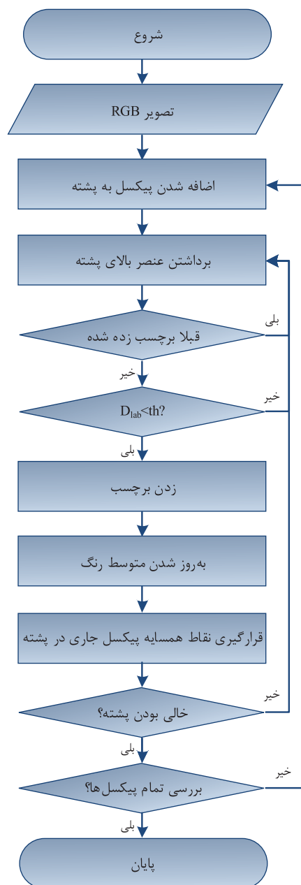
(شکل-۷): روندنامی الگوریتم قطعه بندی پیشنهادی (Figure-7): Flowchart of proposed segmentation algorithm
