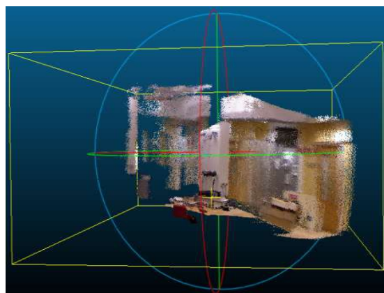
(شکل-۱۵): خروجی الگوریتم ICP روی تمام نقاط (Figure-15): Output of ICP algorithm on all points
