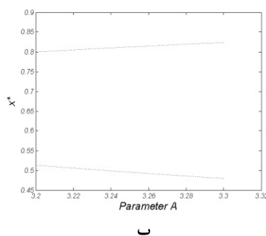
(شکل- ۱): نمودار دوشاخگی لاجستیک ( با
