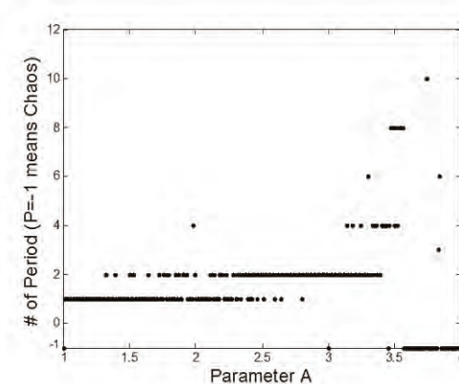
(شکل-۳): نمایش نمودار دوشاخگی
