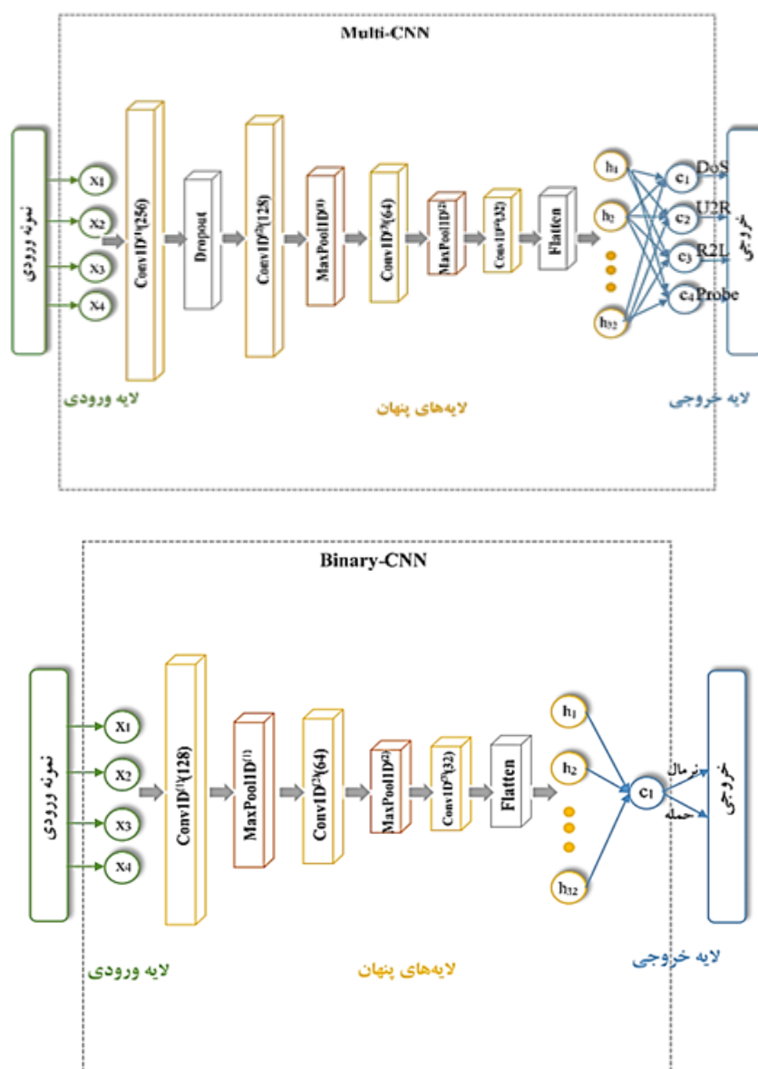
(شکل-۵): معماری شبکه CNN در طبقه‌بندی چندطبقه (Figure-5): Architecture of CNN network in multi-class classification
