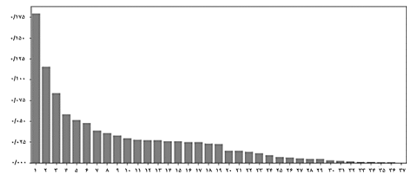
(شکل-۷): نمودار نرخ واریانس بعد از اجرای کاهش بعد PCA
