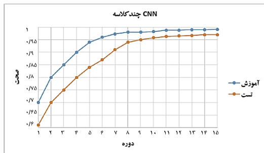
(شکل ۱۱): مقادیر صحت در آموزش و آزمایش CNN چندطبقه
