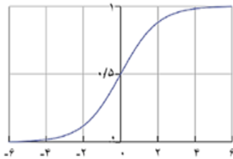
(شکل-۸): نمودار سیگموئید
