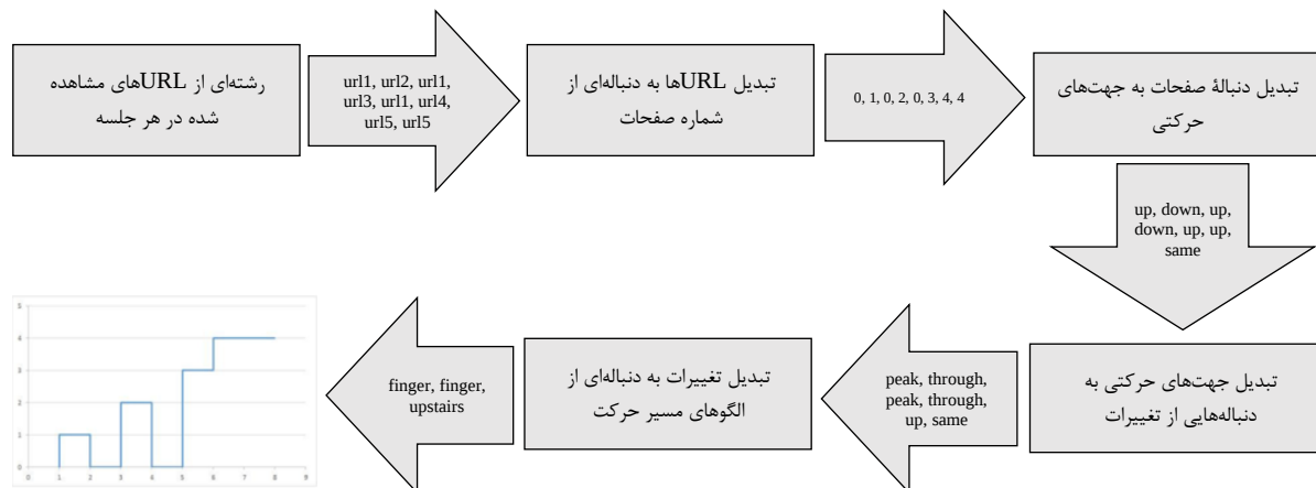
(شکل-۷): روش کشف خودکار الگو (APD) برای تبدیل یک توالی صفحه به نمودار گراف ردپا [ارشته رفتار] (Figure-7): Automatic Pattern Discovery (APD) method for converting a page sequence into a footprint graph [behavior thread]
