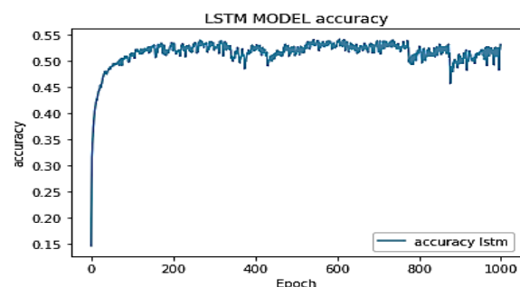
(نمودار ۴-): دقت شبکه LSTM
