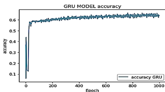
(نمودار-۳): دقت شبکه GRU تک کاربره
