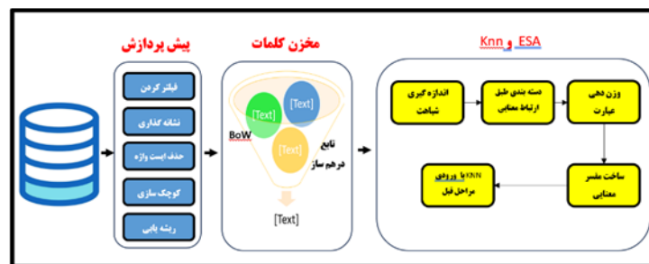
(شکل-۱): مدلی کلی از راه کار پیشنهادی (Figure-1): A general model of the proposed solution
