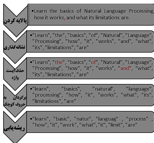
(شکل-۳): مدل پیش پردازش (Figure-2): Pre-processing model
