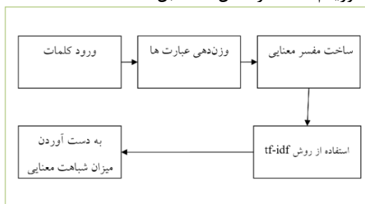
(شکل-۵): روندنمای الگوریتم ESA
