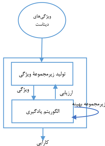
شکل ۲- روند کلی انتخاب ویژگی به روش لفافه Figure 2. Wrapper method procedure
