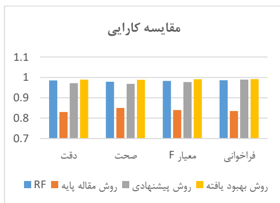
شکل - ۷) مقایسه روش های پیشنهادی و روش ارائه شده در [۲۵]
