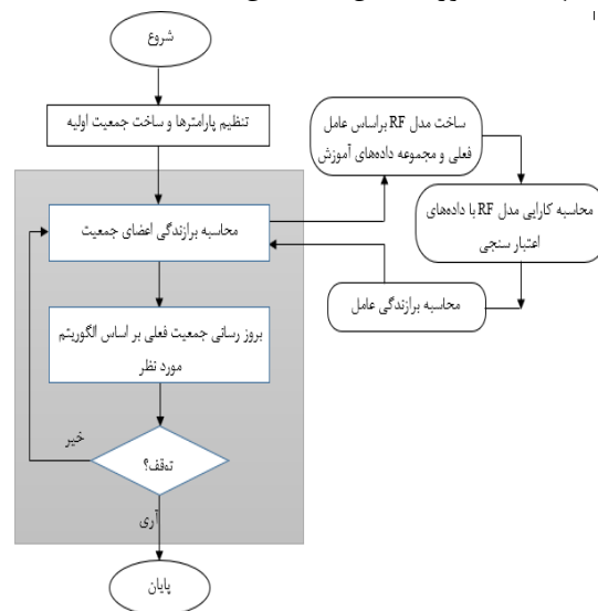
شکل - ۳) روند کلی روش پیشنهادی
