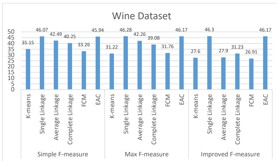
(شکل-۴): اعمال الگوریتم‌های مختلف بر مجموعه داده Wine
