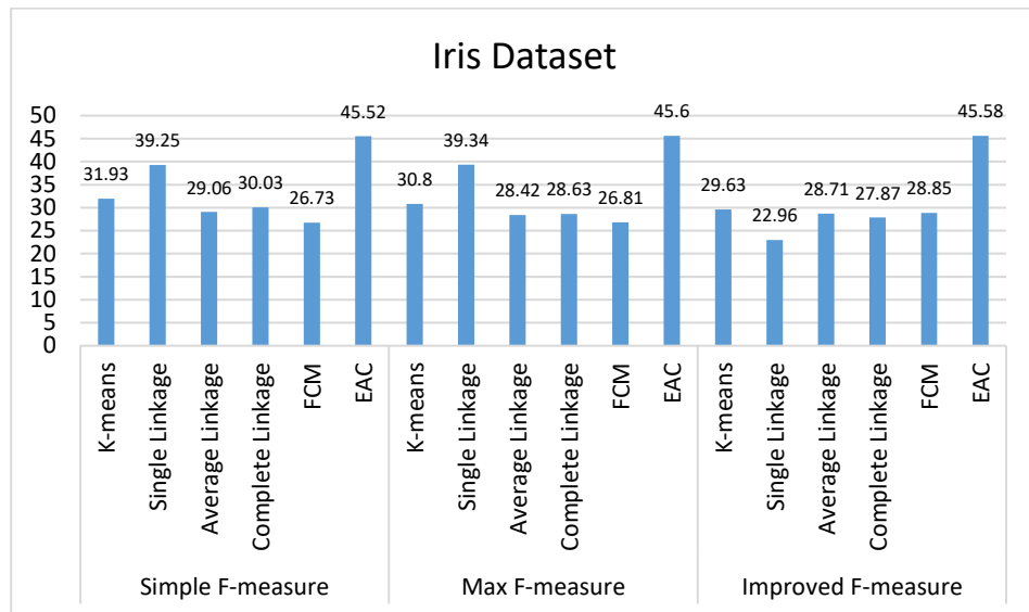
(شکل-۳): اعمال الگوریتم‌های مختلف بر مجموعه داده Iris
