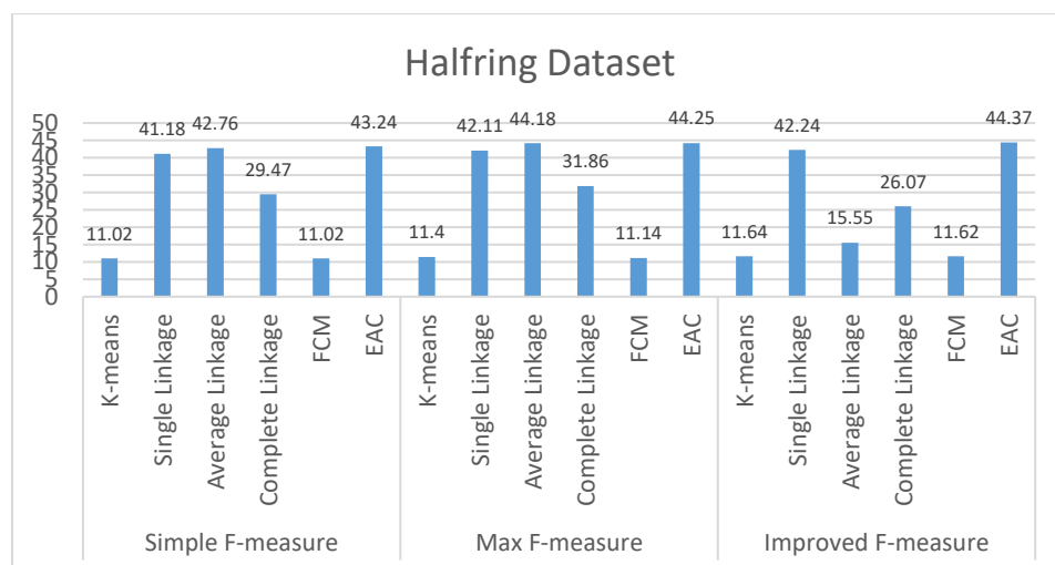
(شکل-۵): اعمال الگوریتم‌های مختلف بر مجموعه داده Halfring
