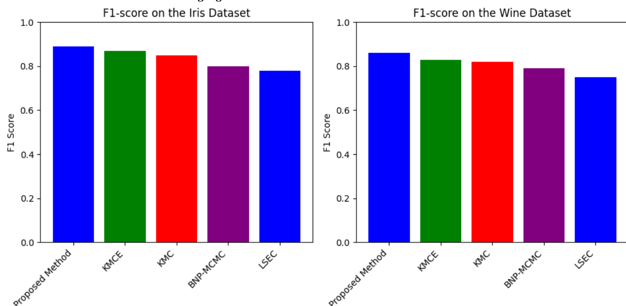
(شکل-۱۱): مقایسه نموداری امتیاز F1 برای روش پیشنهادی در مقابل روش‌های خوشه‌بندی KMCE, KMC, BNP-MCMC, و LSEC
