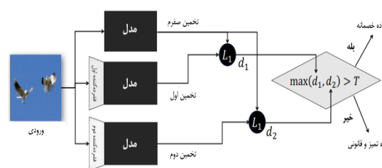
(شکل - ۱۱) - چارچوب تشخیص نمونه خصمانه روش
