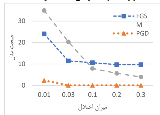
(شکل ۱۹) مقایسه قدرت حملات محصورشده مبتنی بر نرم l_\infty
