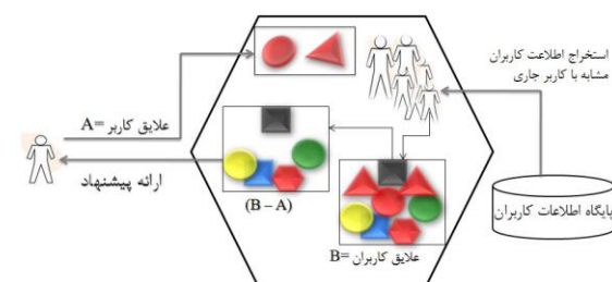
(شکل-۳): روند کار پالایش در الگوریتم مشارکتی (Figure-3): flowchart for the ColF techniques
