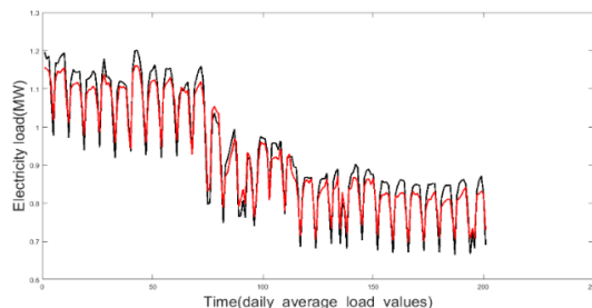
(شکل-۱۵): پیش‌بینی مدل پیشنهادی بار الکتریکی و سیگنال هدف برای داده‌های آزمایشی مجموعه داده لهستان (Figure-15): Predicted the electrical load using the proposed model and the actual load for experimented data Poland data set
