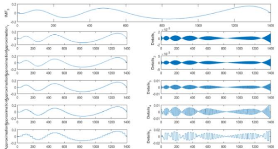
(شکل-۱۰): تقریب و جزئیات مربوط به IMF5
