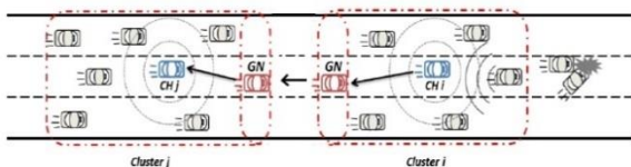
(شکل-۷): نحوه انتشار پیام‌ها در الگوریتم پیشنهادی (Figure-7): Message dissemination in the proposed algorithm
