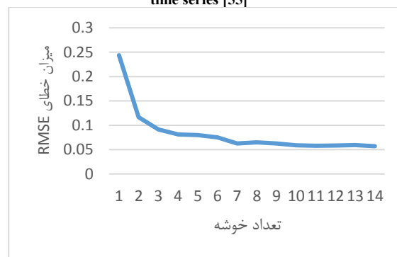
(شکل-۲): تحلیل حساسیت تعداد خوشه بر روی مجموعه داده Energy در درصد گمشده‌گی ۳۰٪ (Figure-2): Sensitivity analysis of the number of clusters on the Energy data set at a missing rate of 30%
