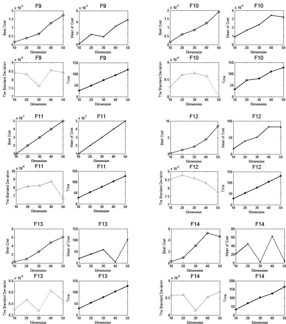
(شکل-۱۱): نمودار بهترین هزینه، میانگین هزینه، انحراف معیار و زمان اجرای الگوریتم‌ها در روش پیشنهادی برای توابع F7 تا F14 میانگین بهترین هزینه الگوریتم‌ها در پنج ابعاد
