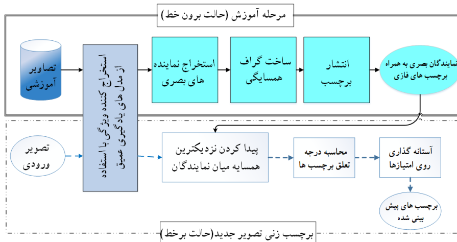
(شکل-۱): روندنمای روش پیشنهادی (Figure-1): Flowdiagram of the proposed method
