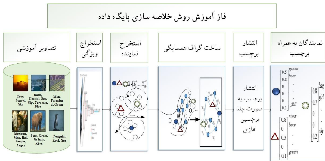
(شکل-۲): فاز خلاصه‌سازی تصاویر آموزشی با روش پیشنهادی (Figure-2): Summarization phase of training images using the proposed method
