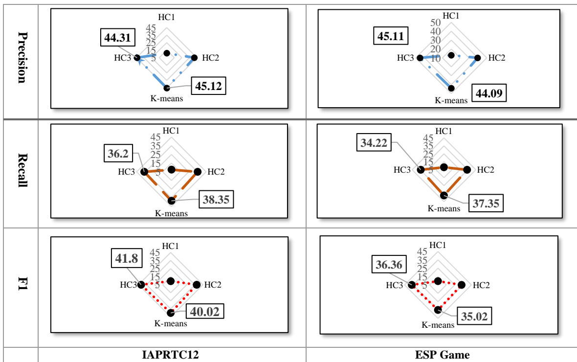
(شکل-۸): مقایسه دو روش استخراج نماینده و تأثیر آن بر روی نتیجه نهایی برچسب‌زنی. هرچه تعداد لایه خوشه‌بندی سلسله مراتبی بیشتر شود، کارایی سامانه نزدیک یا حتی بالاتر از روش خوشه‌بندی رایج خواهد شد. هر ستون مربوط به یک مجموعه داده است.
