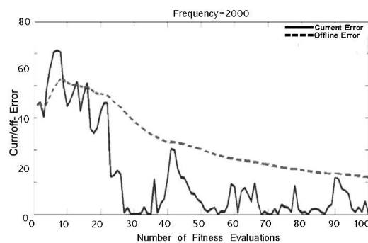
(شکل-۶): نمودار خطای برون خطی و جاری الگوریتم
