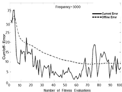
(شکل-۷): نمودار خطای برون خطی و جاری الگوریتم
