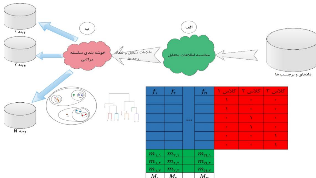
(شکل-۴): مراحل کلی الگوریتم تفکیک خودکار فضای ویژگی
