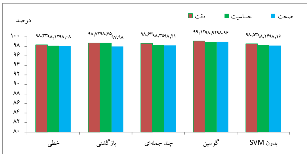
(شکل-۱۵): ارزیابی شاخص دقت، حساسیت و صحت روش پیشنهادی با کرنل های مختلف
