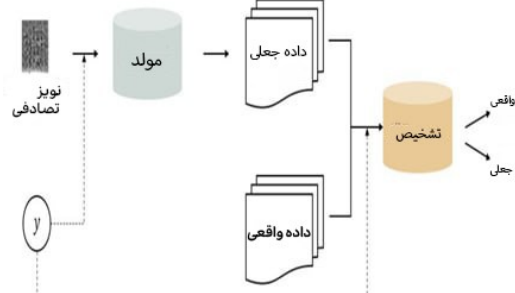
(شکل-۹): عملکرد روش GAN در تولید نمونه‌های مصنوعی برای متعادل‌سازی مجموعه داده [۴۲]
