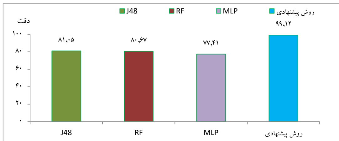
(شکل-۱۶): مقایسه دقت روش پیشنهادی با سه روش یادگیری ماشین
