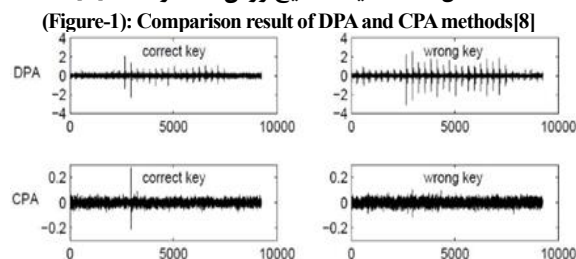
(شکل - ۱): مقایسه نتایج روش CPA و DPA [۸]
