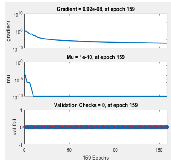
(شکل-۷): خطای رگرسیون در شبکه آموزشی عصبی (Figure-7): Regression Error in Neural Network
