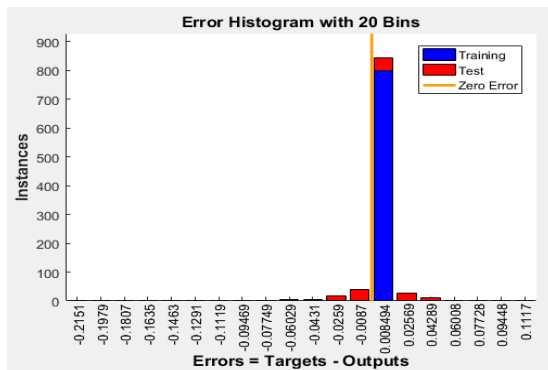
(شکل-۸): خطای بایاس طبیعی شده در شبکه آموزشی عصبی (Figure-8): Error Histogram in neural network
