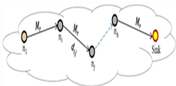
(شکل-۱۲): مسیری با h حسگر رله در روش CDG
