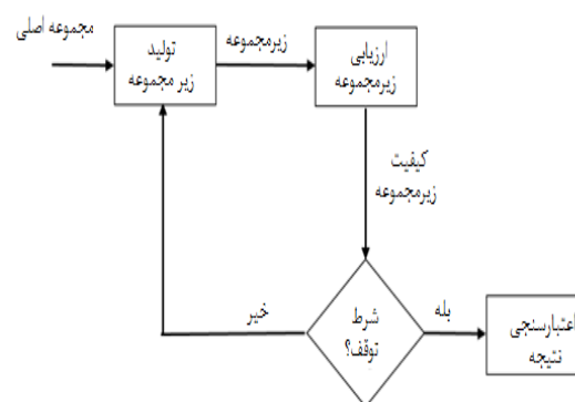
(شکل - ۱) چهار مرحله اساسی در انتخاب ویژگی
