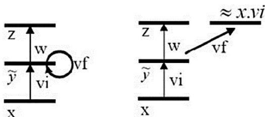
(شکل-۱۱): ساختار یک شبکه عصبی بازگشتی با اتصال
