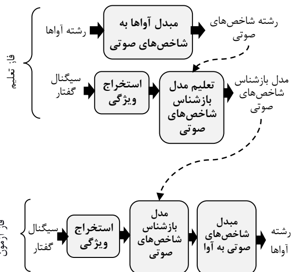
(شکل-۳): سامانه‌ی بازشناسی آوای مبتنی بر شاخص‌های صوتی.
