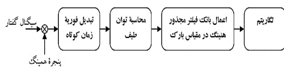
(شکل-۱۳): روش استخراج LHCB [۳]. (Figure-13): LHCB extraction method [3].
