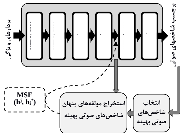
(شکل-۱۲): طرح ۴ جبران‌سازی- شکل‌دهی مؤلفه‌های
