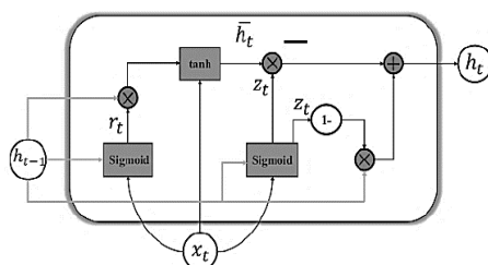
(شکل ۴-۴): ساختار GRU (Figure-4): The structure of GRU
