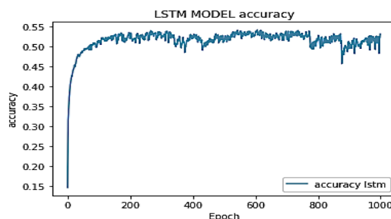
(نمودار-۴): دقت شبکه LSTM (Chart-4): Accuracy of LSTM network
