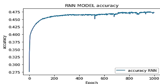
(نمودار-۵): دقت شبکه RNN (Chart-5): Accuracy of RNN network
