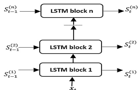
(شکل ۳-۳): معماری شبکه LSTM عمیق (Figure-3): Deep LSTM network architecture
