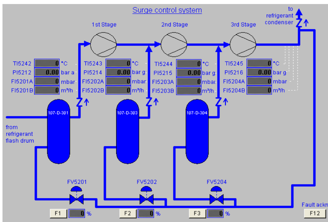
(شکل-۱): سامانه کنترل سرج کمپرسور مورد مطالعه (Figure- 1): Surge control system of compressor
