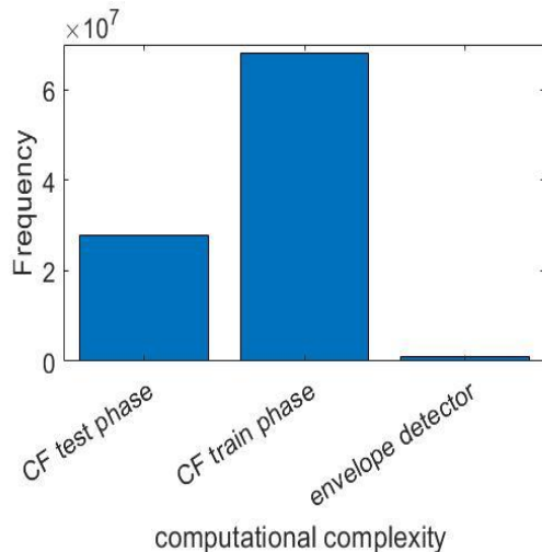
(شکل-۲۳): هیستوگرام مقایسه میزان پیچیدگی روش پیشنهادی و روش آشکارساز پوش (Figure-23): Computational complexity of the proposed detector and envelope detector
