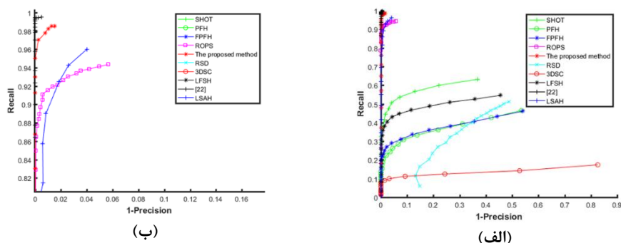
(شکل-۶): الف) نتایج RPC مربوط به تمامی توصیف گرها، ب) شکل بزرگ شده الف) برای وضوح بیشتر (Figure-6): The RPC-based evaluation of the descriptors
