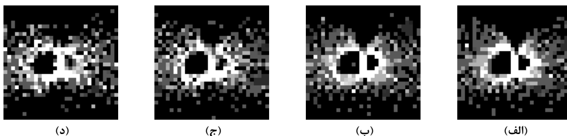
(شکل-۷): ویژگی‌های به دست آمده برای یک نقطه، الف) در صحنه بدون نویز و صحنه‌های با نویز گوسی با انحراف معیار (ب) ۰/۱ وضوح مش، (ج) ۰/۳ وضوح مش، و (د) ۰/۵ وضوح مش (Figure-7): Achieved features for a point in (a) the noise-free scene, the scenes with standard deviation (b) 0.1 mr, (c) 0.3 mr, and (d) 0.5 mr
