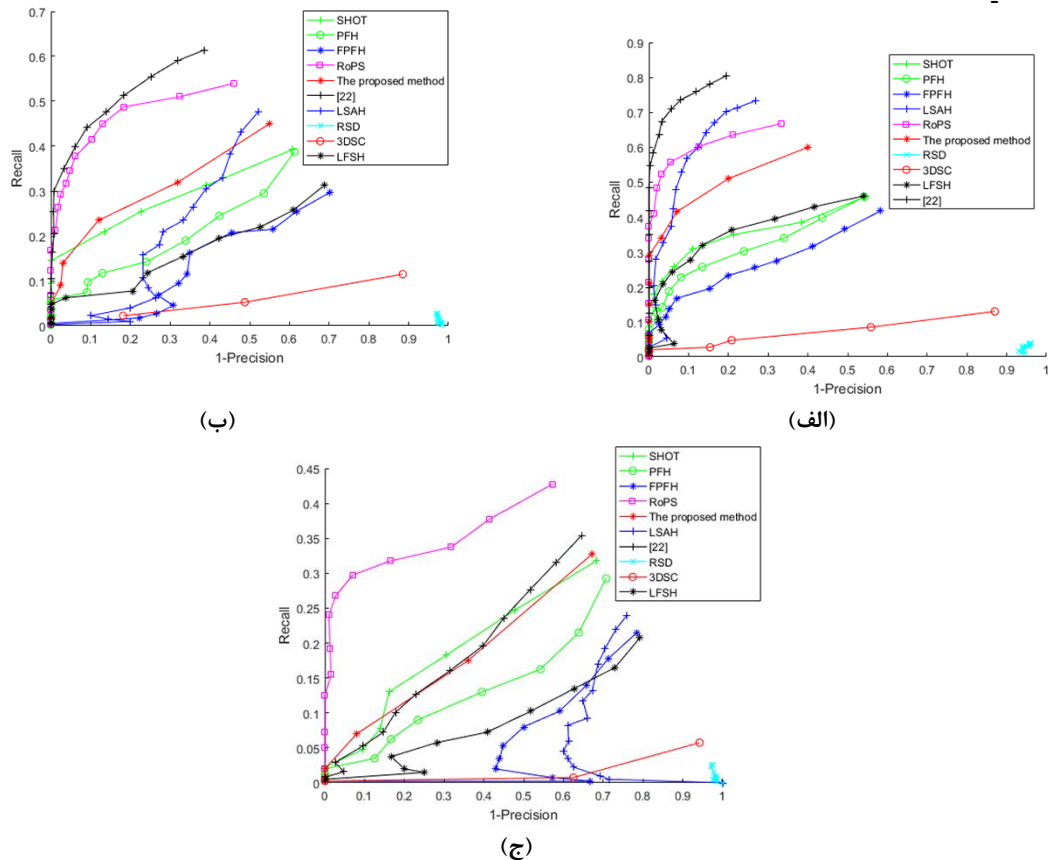
(شکل-۱۰): نتایج RPC مربوط به تمامی توصیف‌گرها در سطوح مختلف مش رزولوشن با فاکتورهای کاهش \frac{1}{8} (الف) \frac{1}{4} (ب) \frac{1}{2} (ج)
