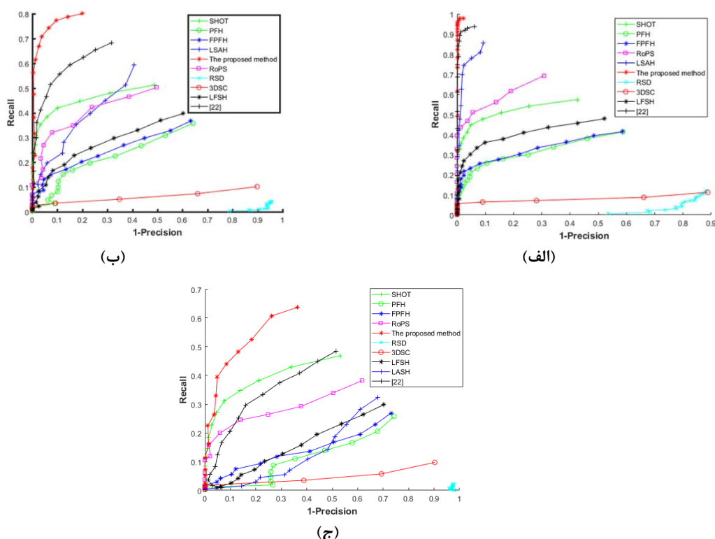
(شکل-۸): نتایج RPC مربوط به تمامی توصیف گرها در سطوح مختلف نویز گوسی با انحراف معیار الف) ۰/۱ وضوح مش، (ب) ۰/۳ وضوح مش، و (ج) ۰/۵ وضوح مش
